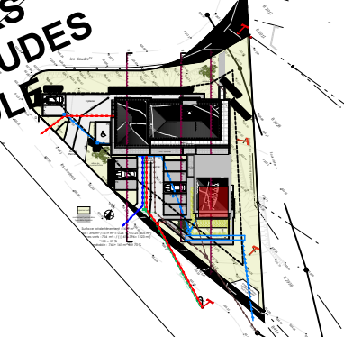
Plan de masse - situation niveau Rez de chaussée bas
